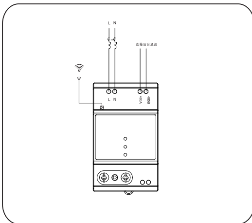
接线图
